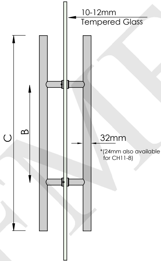
ELEVATION
